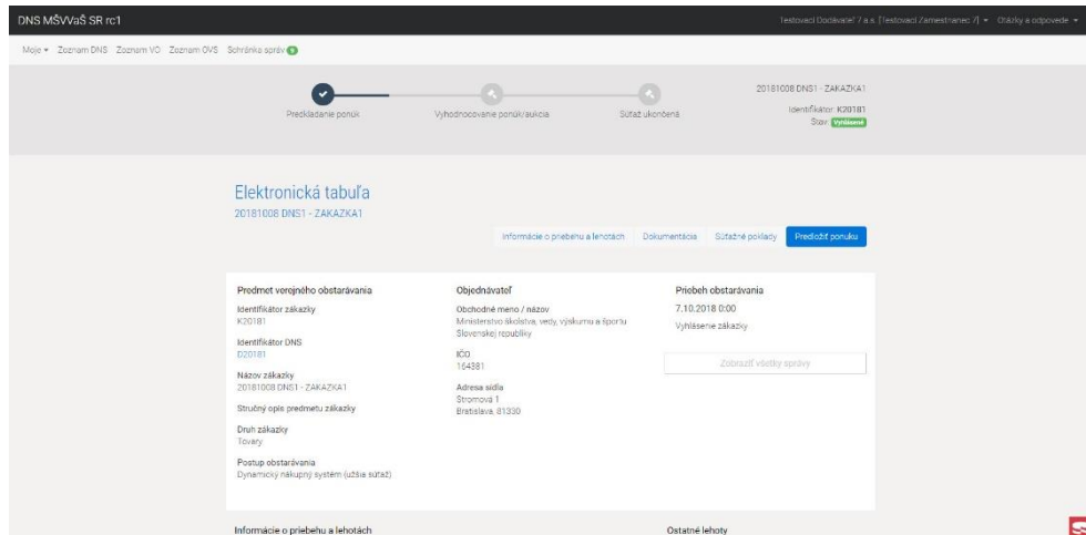
Obrázok 4: Elektronická tabuľa
