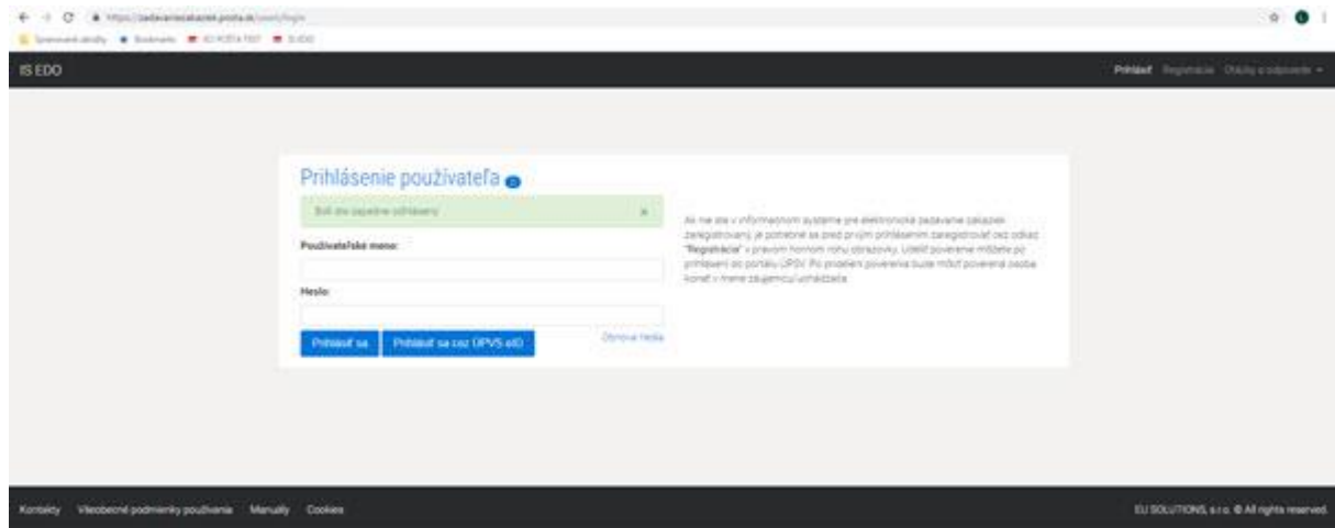
Obrázok 1: Prihlasovacia obrazovka
